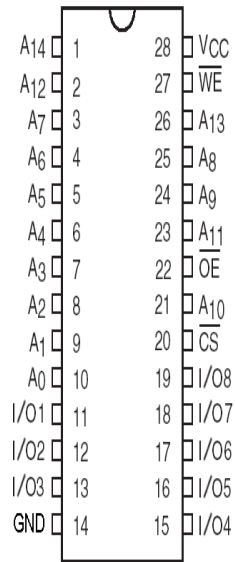
28-Pin DIP Module
